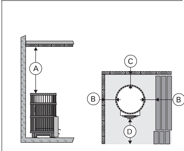
Figure 9. Safety distances (all dimensions in millimeters) Abbildung 9. Sicherheitsabstände (alle Abmessungen in Millimetern)
